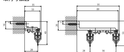
取付寸法図
