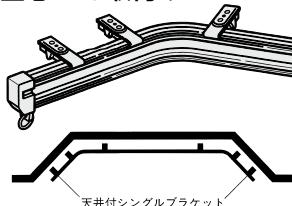
出窓への取付け
