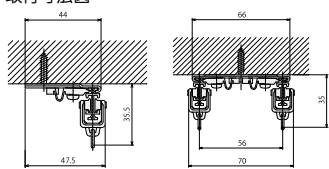
取付寸法図
