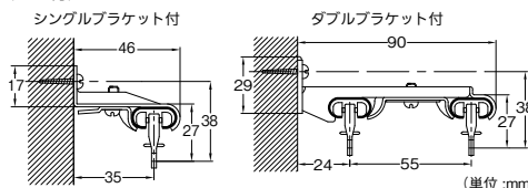
取付寸法図 (正面付)
